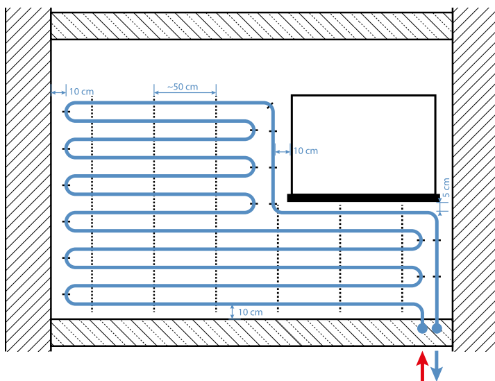
Rys. 34. Odległości montażowe w ogrzewaniu ściennym.
