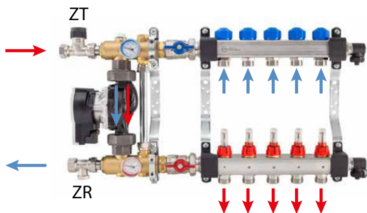
Rys. 55. Rozdzielacz z układem mieszającym USFP – kierunki przepływów.
