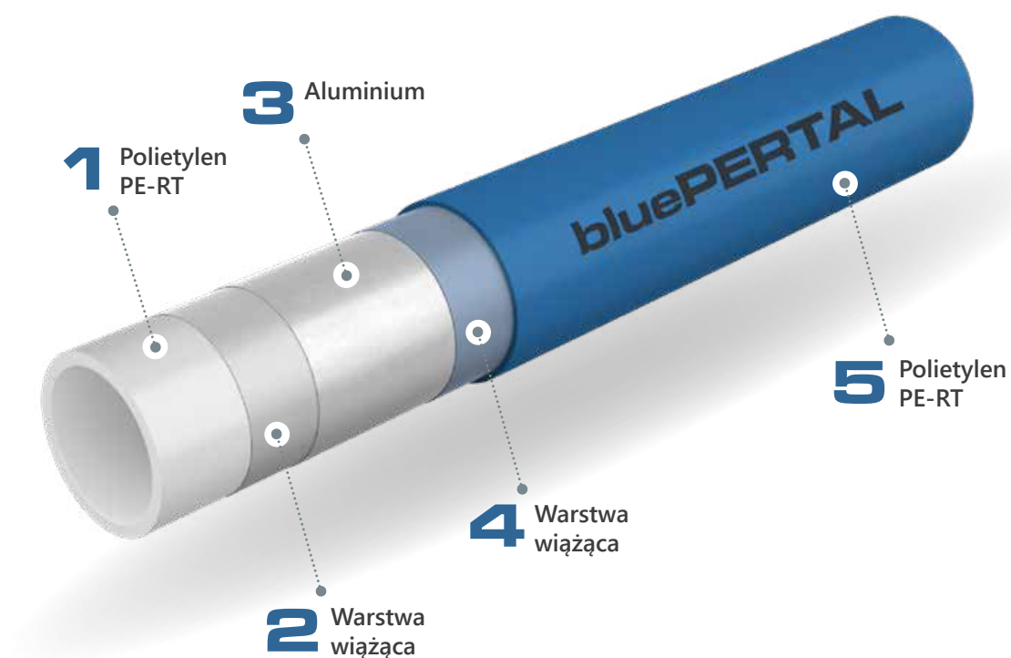
Rys. 46. Budwa rury bluePERTAL z warstwą aluminium.
