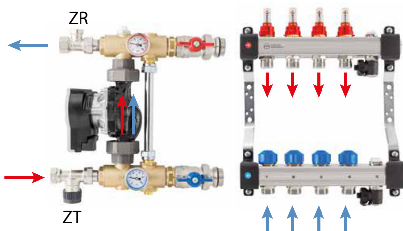
Rys. 56. Grupa pompowa stałowartościowa z rozdzielaczem UFST – kierunki przepływów.
