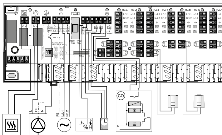
Rys. 68. Konfiguracja listwy elektrycznej Basic+ 230 V lub 24 V z modułem pompowym, modułem kotła i urządzeniami peryferyjnymi.
