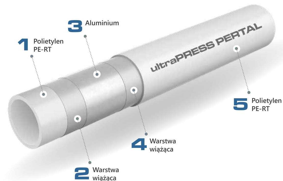
Rys. 47. Budowa rur PERTAL KAN-therm z warstwą aluminium.
