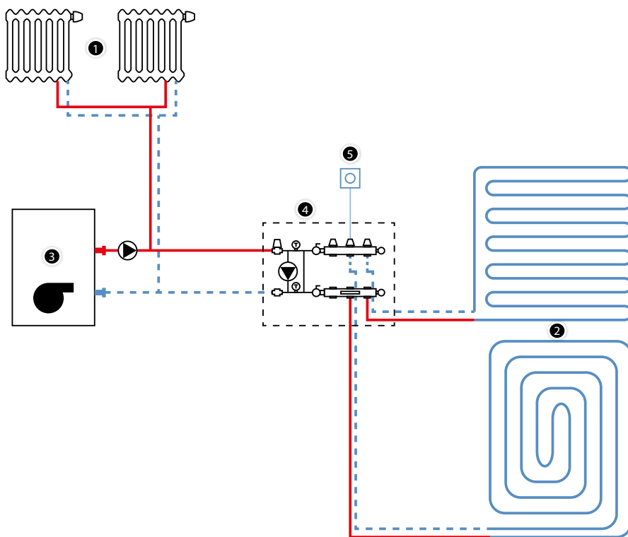
Rys. 54. Miejskowy układ zmieszania.
